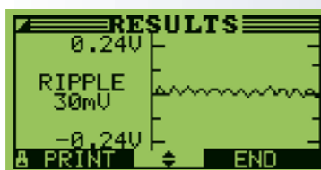
Testresultat för laddningssystem, rippelström
